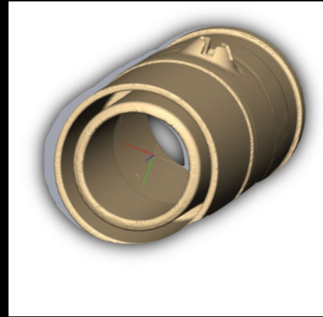
Falfiau allanadlu 3D wedi'u hargraffu Enghraifft o ailbwrpasu cyfarpar er mwyn bodloni gofynion newydd
